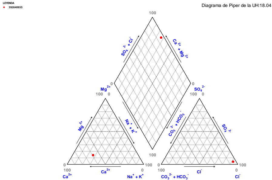
Diagrama de Piper de la UH 18.04 (octubre de 2008)
