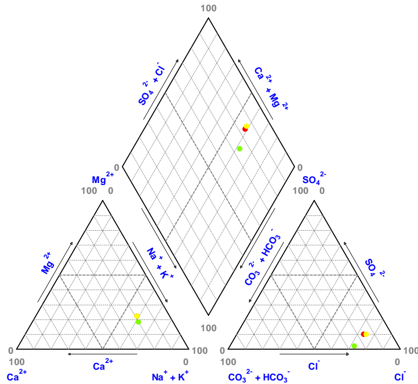
Diagrama de Piper de la UH:18.20
