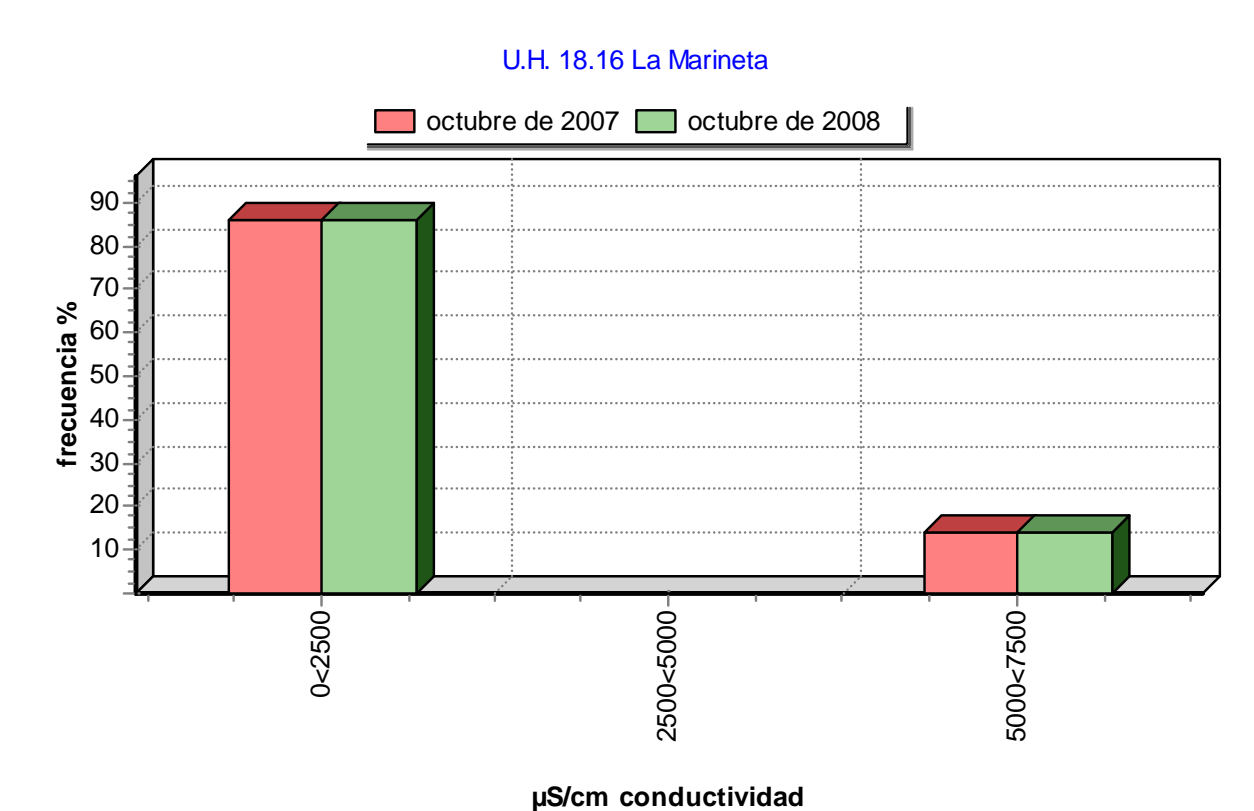
Gráfica de frecuencias de conductividad de la UH 18.16
