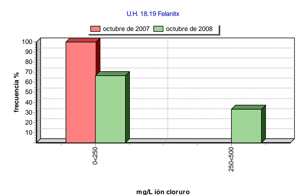
Gráfica de frecuencias de ión cloruro de la UH 18.19
