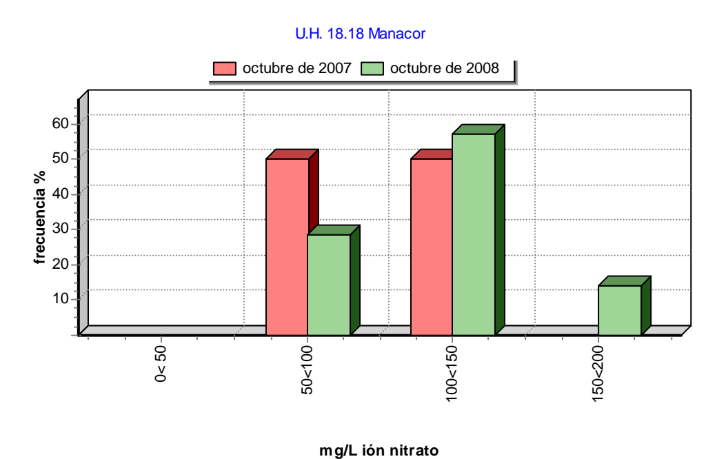
Gráfica de frecuencias de ión nitrato de la UH 18.18
