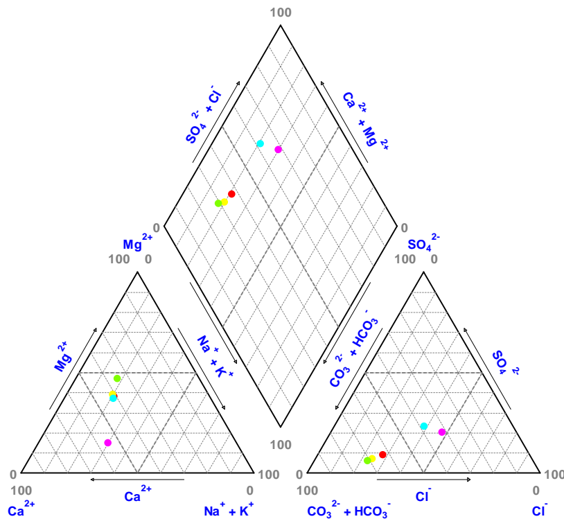
Diagrama de Piper de la UH:18.19
