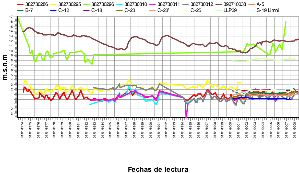
Evolución piezométrica de la U.H. 18.14 - Pla de Palma
