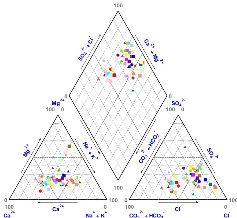
Diagrama de Piper de la UH:18.11
