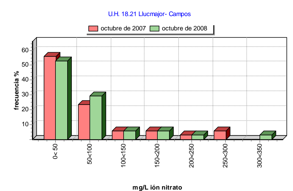
Gráfica de frecuencias de ión nitrato de la UH 18.21
