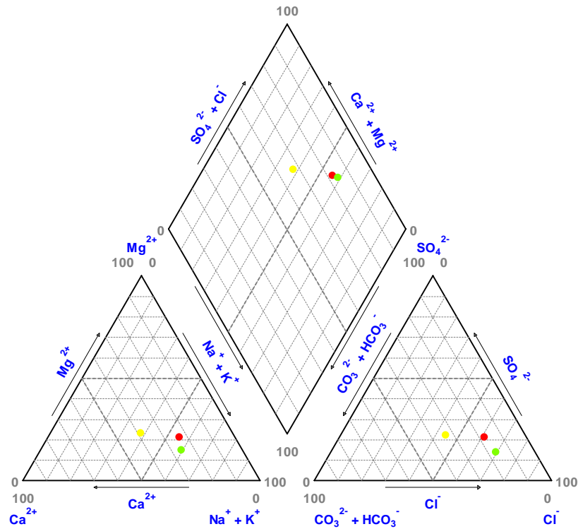
Diagrama de Piper de la UH:18.13
