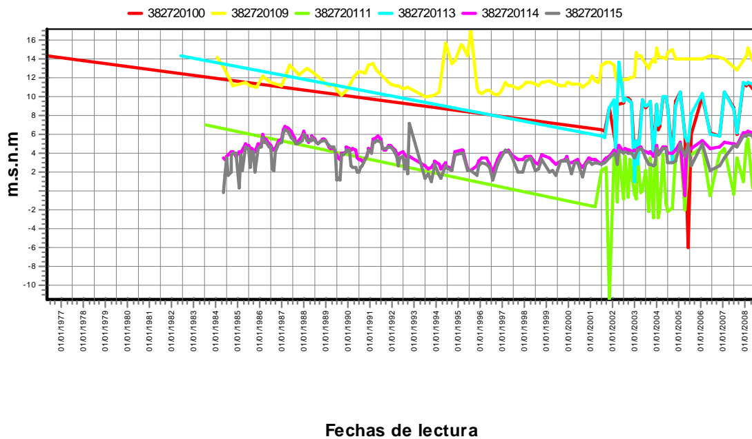
Evolución piezométrica de la U.H. 18.13 - Na Burguesa
