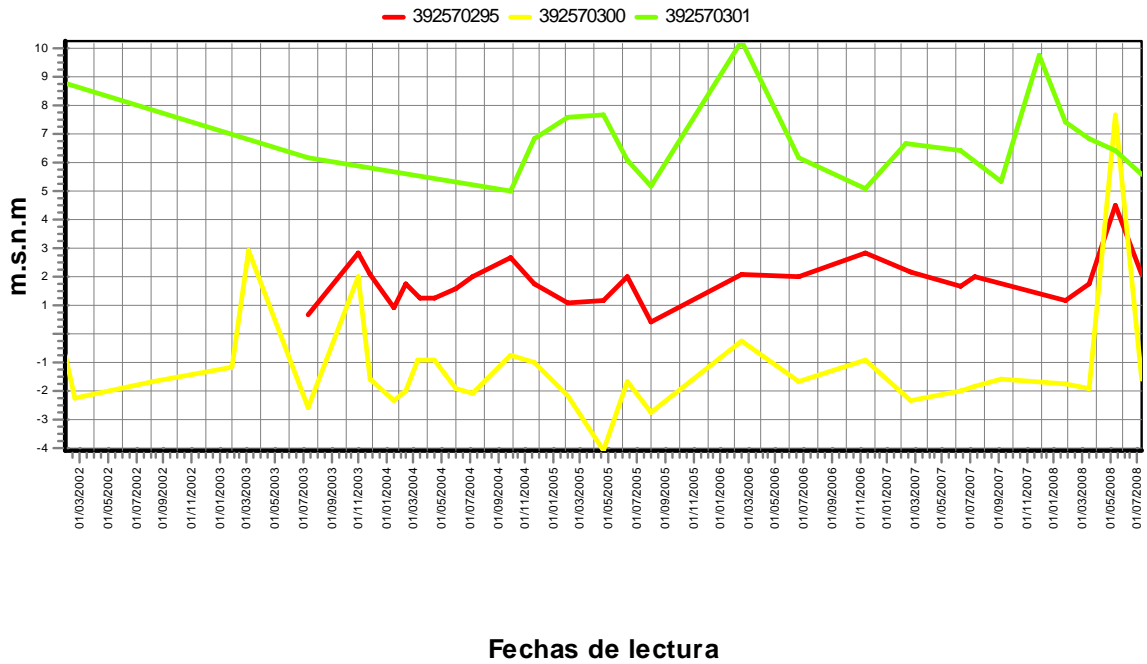
Evolución piezométrica de la U.H. 18.04 - Formentor
