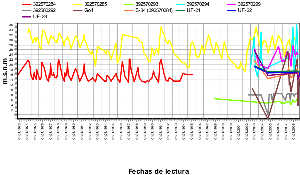
Evolución piezométrica de la U.H. 18.05 - Almadrava
