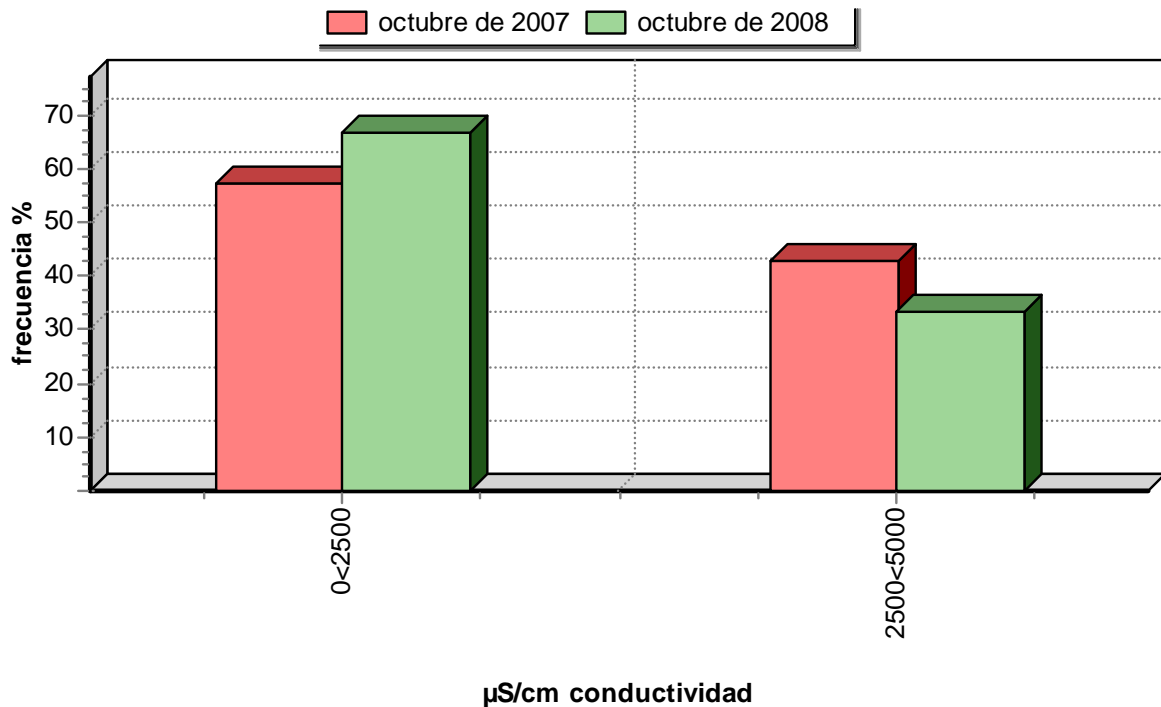
Gráfica de frecuencias de conductividad de la UH 18.12
