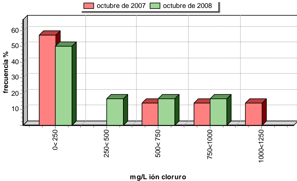
Gráfica de frecuencias de ión cloruro de la UH 18.12
