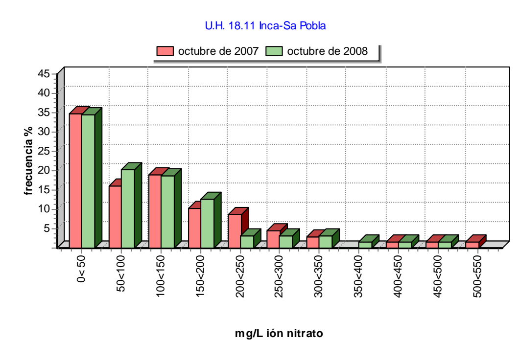
Gráfica de frecuencias de ión nitrato de la UH 18.11
