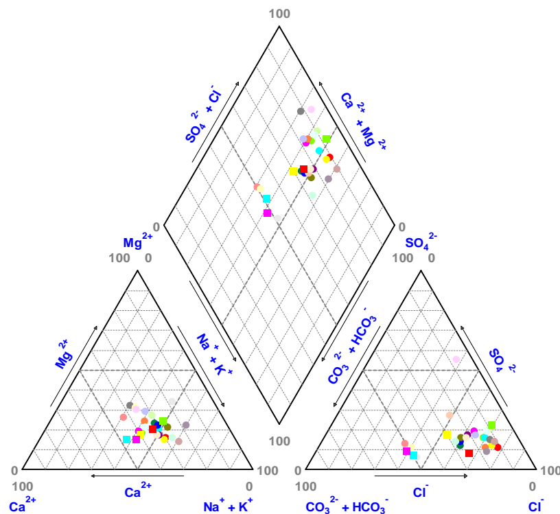
Diagrama de Piper de la UH:18.14
