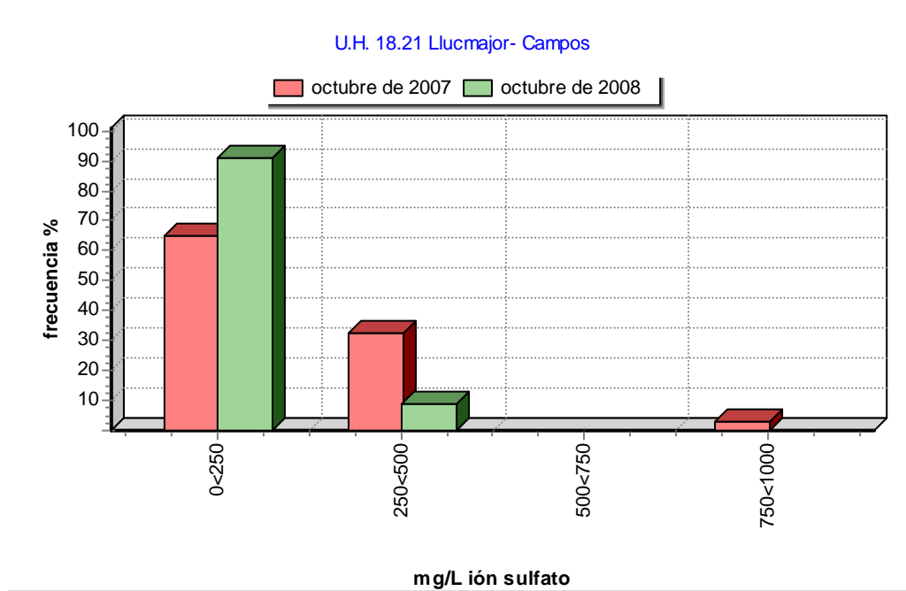
Gráfica de frecuencias de ión sulfato de la UH 18.21
