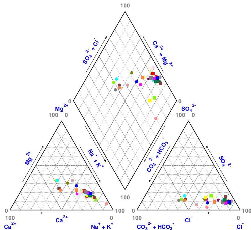
Diagrama de Piper de la UH:18.21
