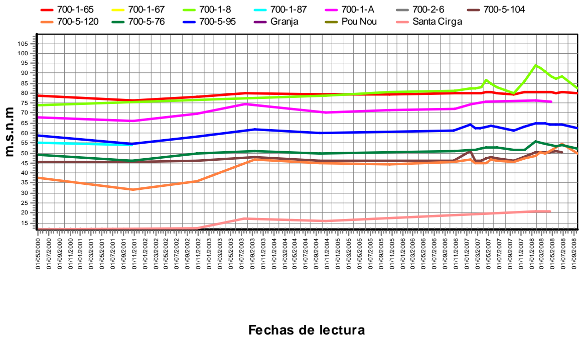
Evolución piezométrica de la U.H. 18.18 - Manacor
