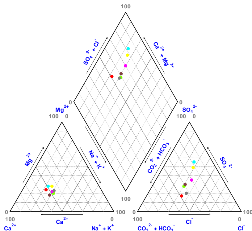
Diagrama de Piper de la UH:18.01
